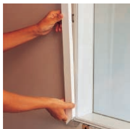
Set costruttivo per vetrate prefabbricate su pareti leggere Knauf
